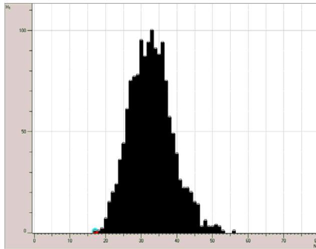
Fig.1 Distribuția Poisson – histograma (construită cu softul CASYY Lab)
