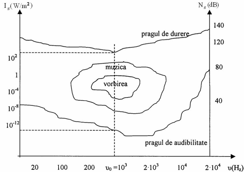
Fig. V.1. Pragul de audibilitate și pragul de durere în funcție de frecvența sunetului.
